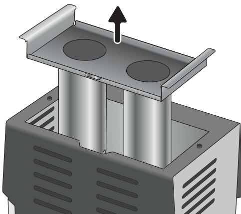
Abb. 4: Rösteinsatz ausbauen
