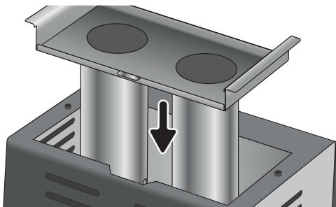
Abb. 9: Rösteinsatz korrekt einsetzen
