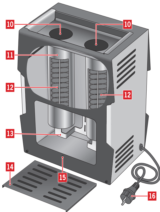
Abb. 2: Rückansicht und Innenleben (Schnittdarstellung)
