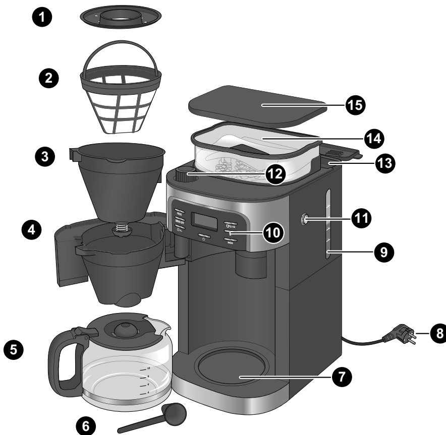
Abb. 1: Apparatets dele
